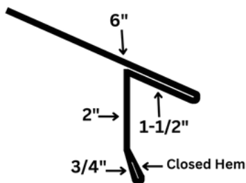
SS200 DRIP EDGE
